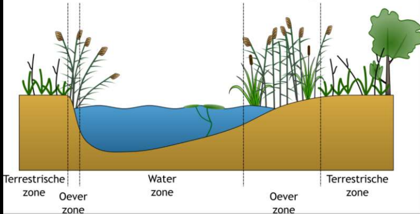
Figuur 2. Voorbeeld en schematische weergave van een natuurvriendelijke oever (NVO) en een steile oever(referentie).
